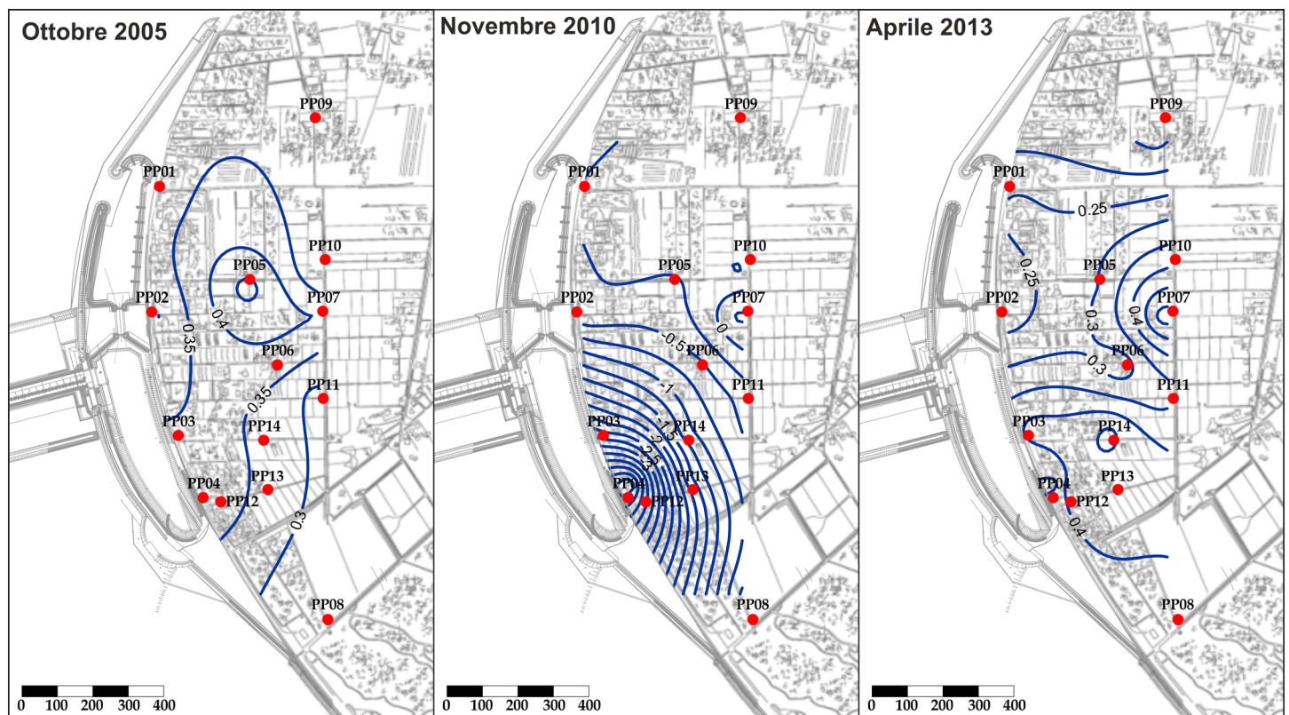
Confronto tra le curve di livello (piezometrie) di falda profonda prima del pompaggio di cantiere (Ottobre 2005), durante il pompaggio (Novembre 2010) e dopo il termine del pompaggio (Aprile 2013). In rosso sono indicati i piezometri profondi (PP01÷14) dai quali sono stati tratti i dati puntuali di carico idraulico della falda.
