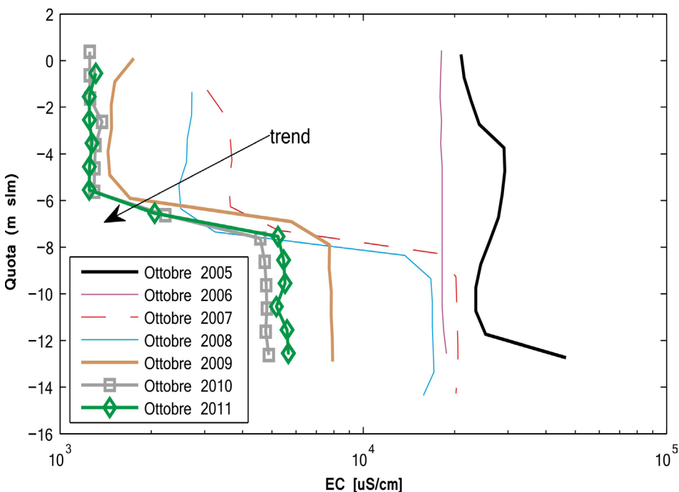
Profili verticali di conducibilità elettrica nel piezometro PS04, vicino al bacino di prefabbricazione delle barriere mobili. Si osserva che, nel tempo, la conducibilità (e quindi la salinità) dell'acqua si è notevolmente ridotta.
