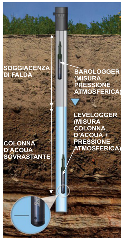
Schema di installazione e grandezze misurate dagli strumenti installati nei piezometri (Levellogger e dai Barologger).
