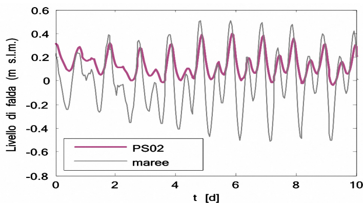
Dinamica dei livelli in un piezometro lungo la costa (PS02, a circa 20 m dalla costa).
