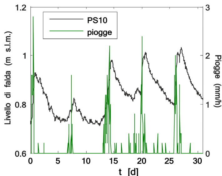
Dinamica dei livelli in un piezometro nell'entroterra (PS10, a 500 m dalla costa).
