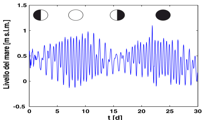
Andamento delle maree secondo le fasi lunari: primo quarto, luna piena, ultimo quarto, luna nuova.
