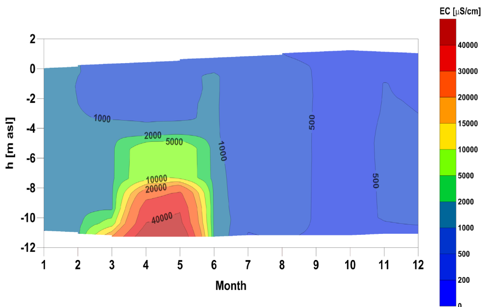
Grafico che evidenzia come varia, nel corso delle stagioni, l'andamento verticale della conducibilità elettrica e quindi della salinità dell'acqua in un piezometro dell'acquifero superficiale (PS06). Si osserva come in estate si verifichi un netto incremento dei valori.
